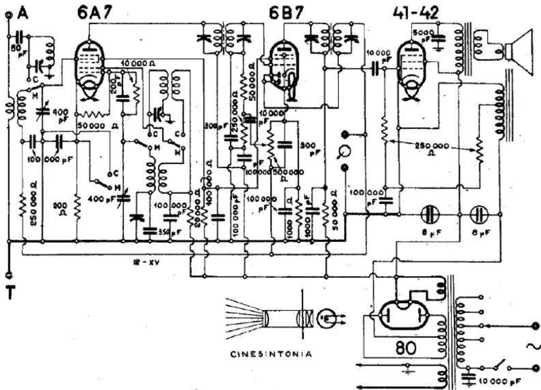
AREL - MODD. « 4 VALVOLE » - « PRODIGIO »
